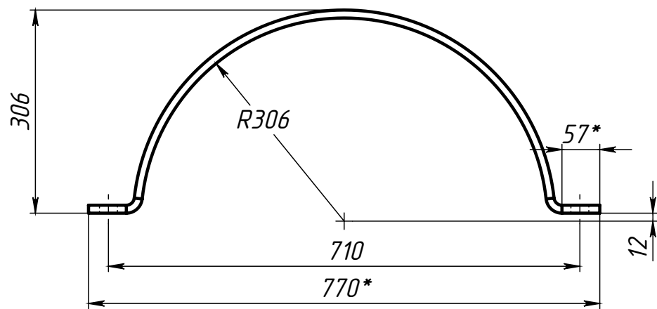
Поз.4 (Полухомут)
